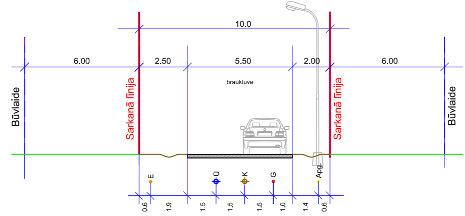
ŠĶĒRSPROFILS 10 m
