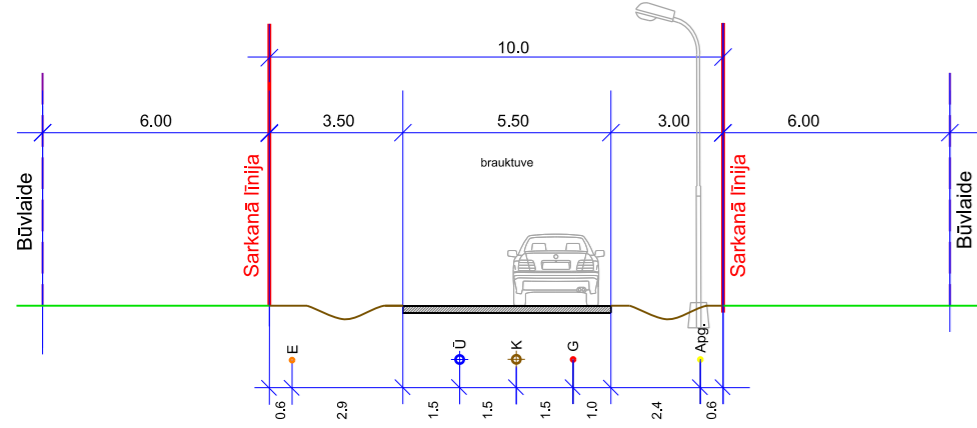
ŠĶĒRSPROFILS 12 m
