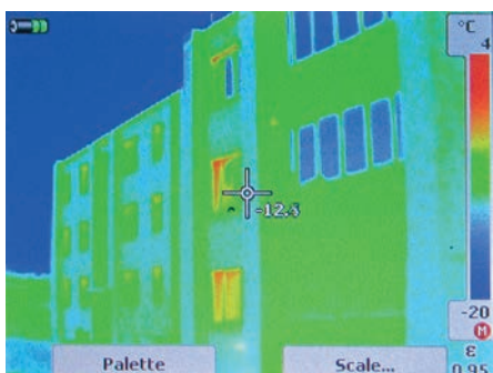
Termogrāfa uzņēmumi pie nosiltinātas ēkas Pirmā ielā 32, Ādažos
