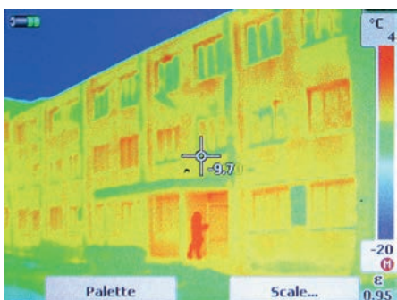
Termogrāfa uzņēmumi pie nenosiltinātām ēkām, Pirmā ielā 34 un Pirmā ielā 27, Ādažos
