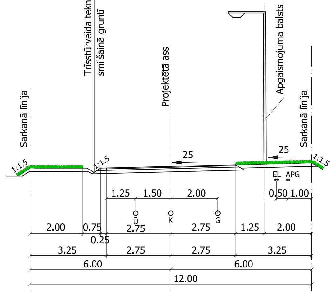
Pamatprofils pie sarkanā līniju platuma 12.0m* A-A, B-B, C-C, D-D, E-E M1:100
