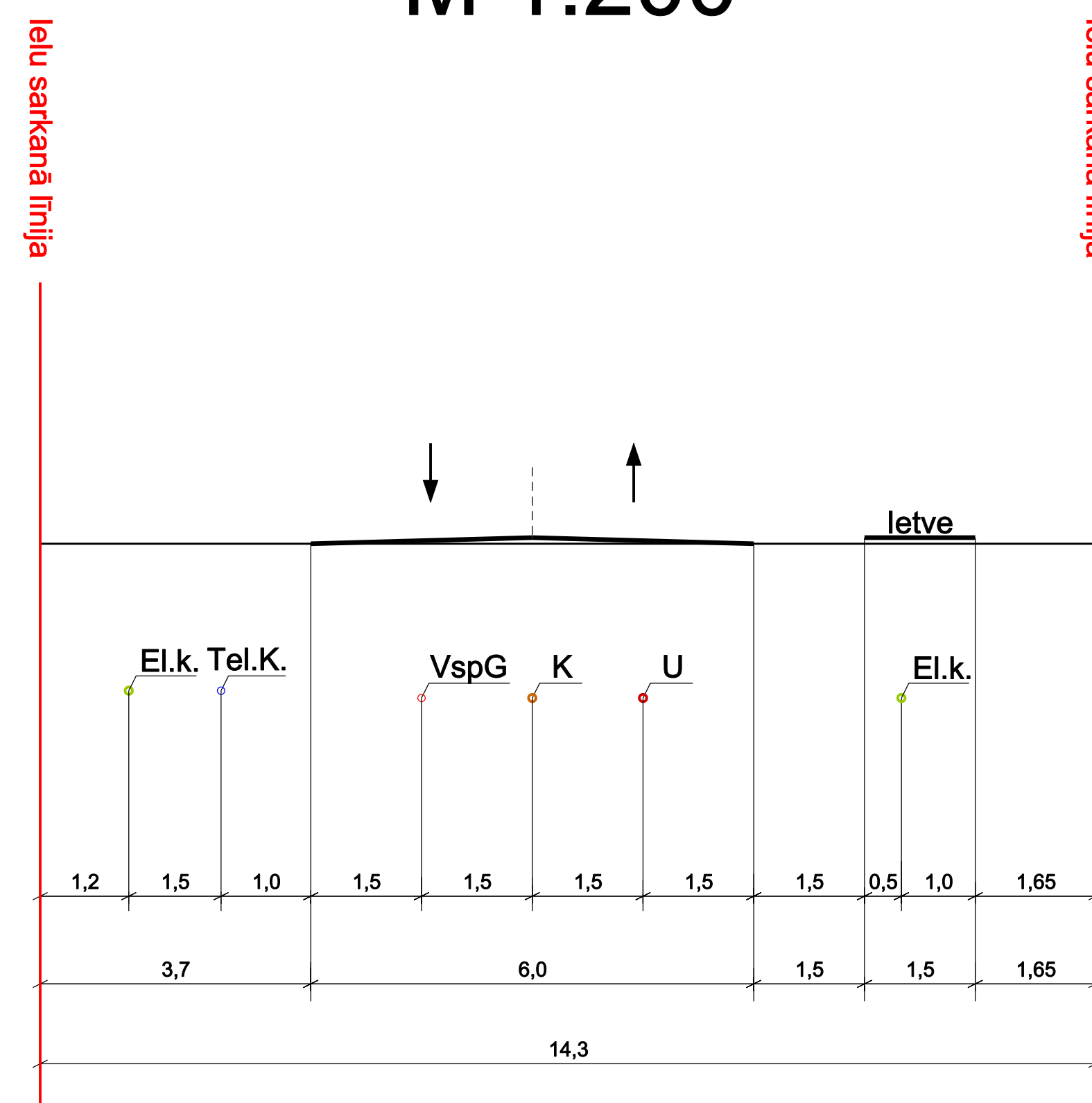
Ielas griezumums A-A M 1:200
